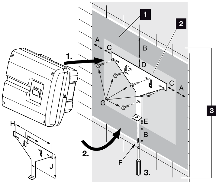
Fig. 19: Montering på væggen vha. vægholder
