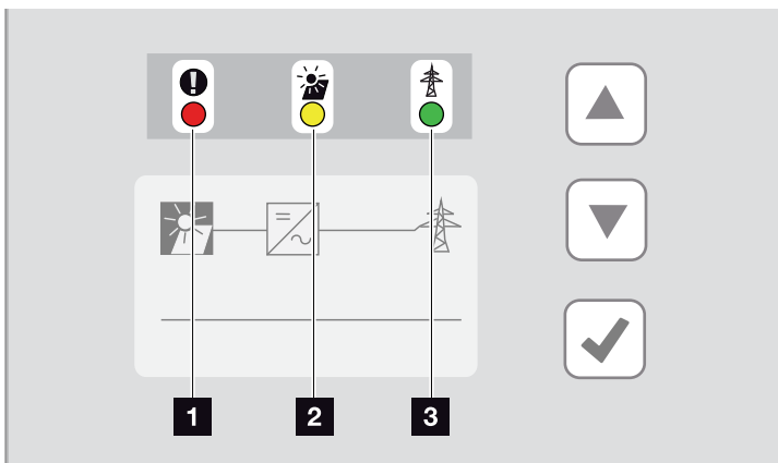
Fig. 41: LED'er på vekselstrømsomformerens display
