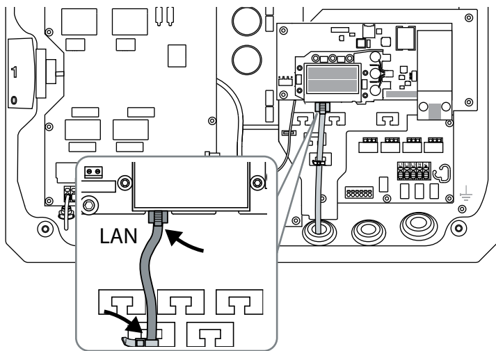
Fig. 67: Tilslutningsklemme elmåler
