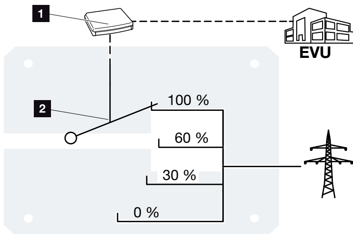
Fig. 50: Styring af virkeeffekten med en fjernovervågningsmodtager
