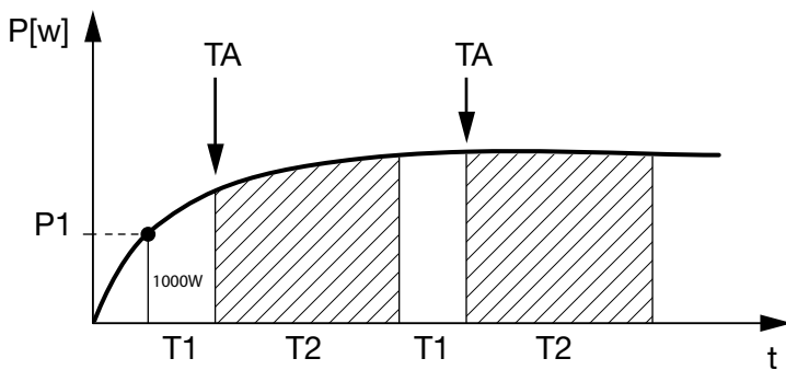
Fig. 56: Kurve egetforbrug (funktion 1) uden strømsensor
