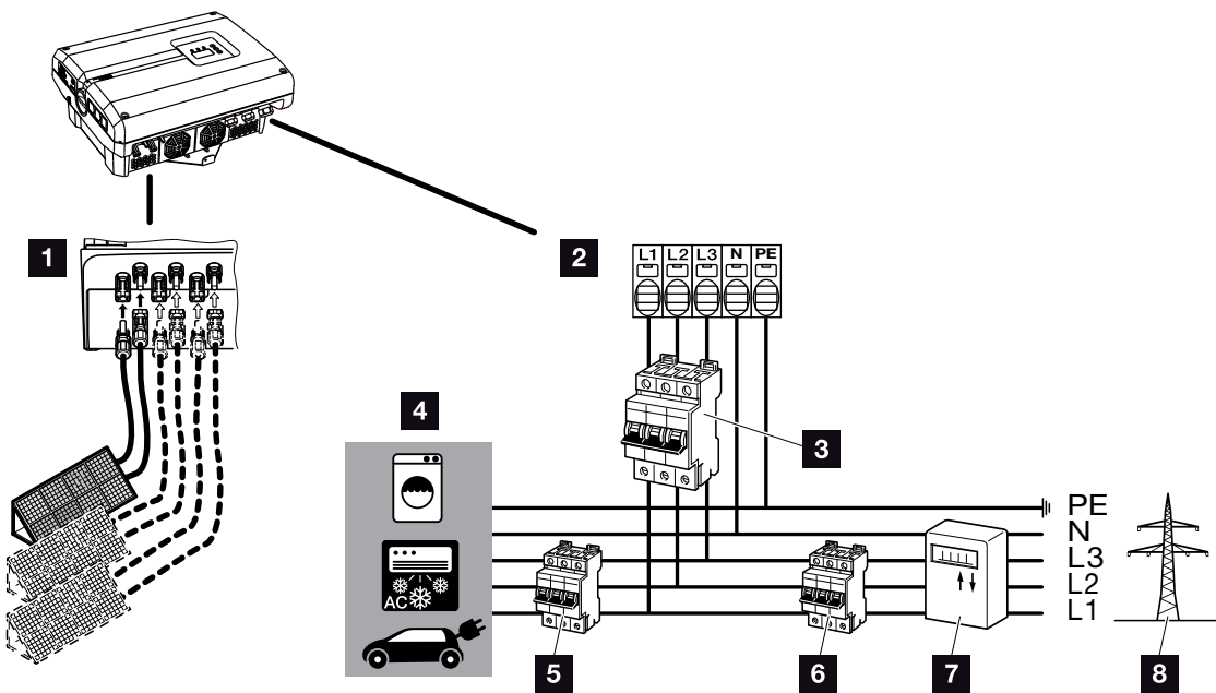
Fig. 21: Oversigt over de elektriske tilslutninger
