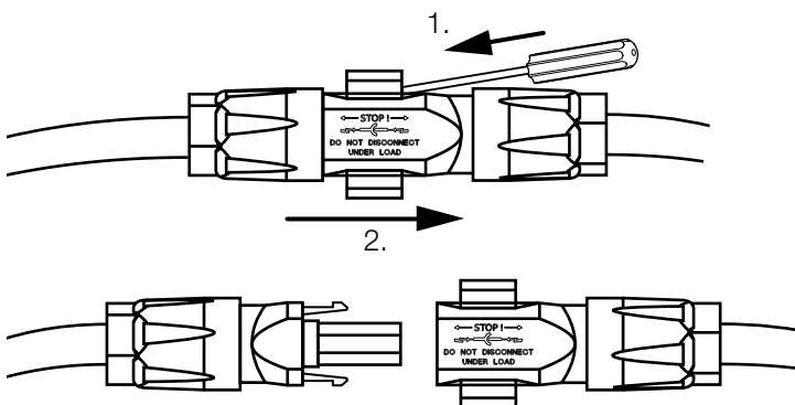
Fig. 37: Tag SUNCLIX stikket ud
