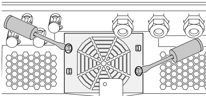
Fig. 61: Løsn fastgørelseslaskerne
