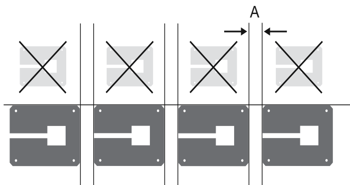
Fig. 20: Montering på væg af flere vekselstrømsomformere
