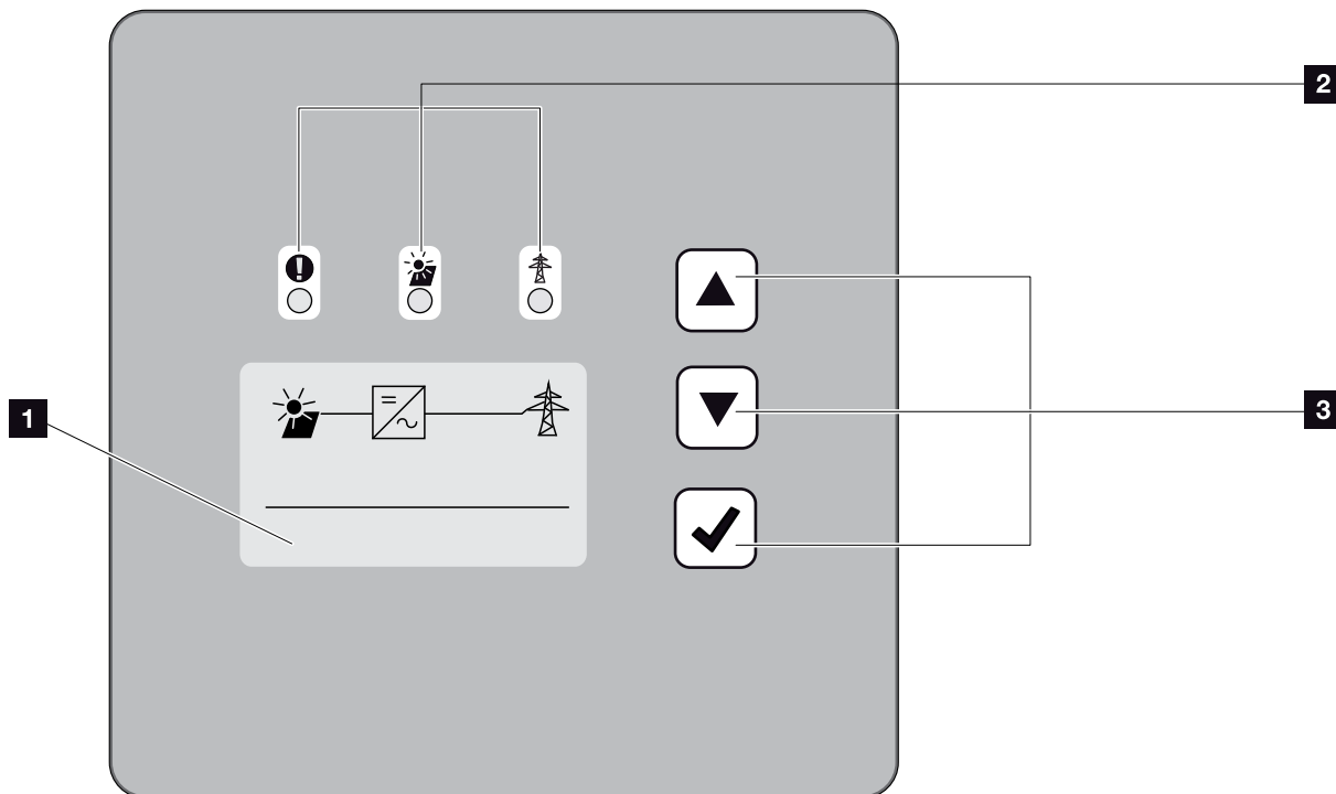
Fig. 15: Betjeningsfelt
