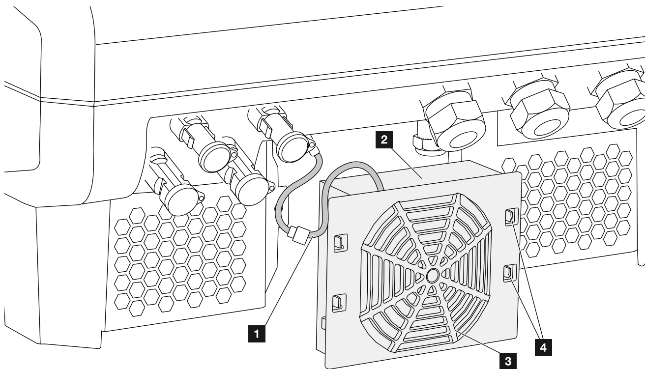
Fig. 59: Afmontering af ventilator, oversigt
