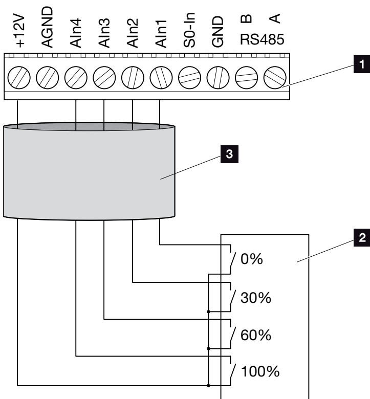
Fig. 52: Tilslutning fjernovervågningsmodtager
