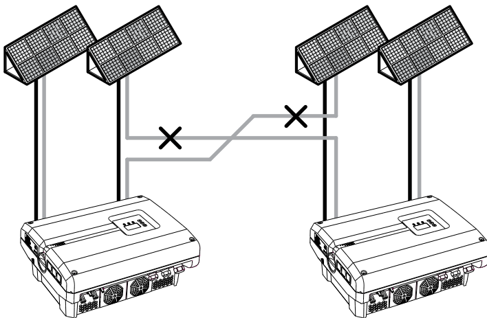
Fig. 29: Forkert bestykning FV-generatorer
