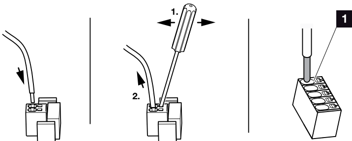
Fig. 23: Fjederbelastet klemrække
