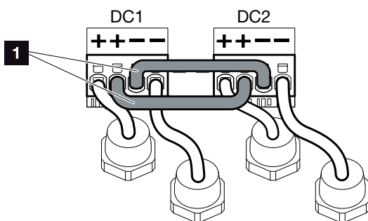
Fig. 28: Indgang 1 og 2 er parallelforbundet
