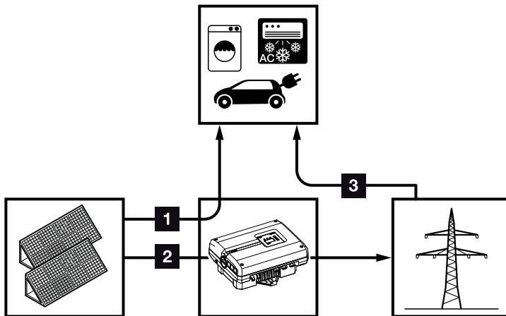
Fig. 43: Styring og fordeling af energistrømmene
