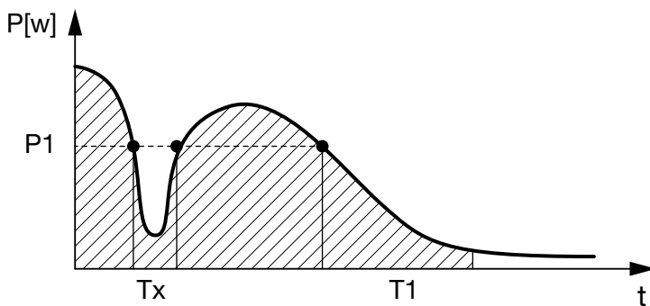
Fig. 58: Kort forsinkelse ved effektreduktion/forstyrrelse
