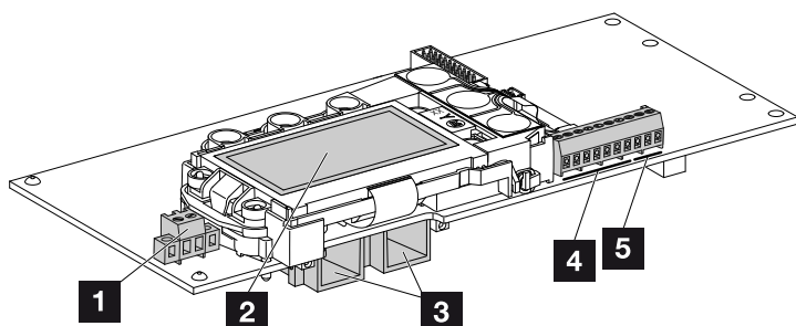
Fig. 14: Kommunikationsboardets komponenter
