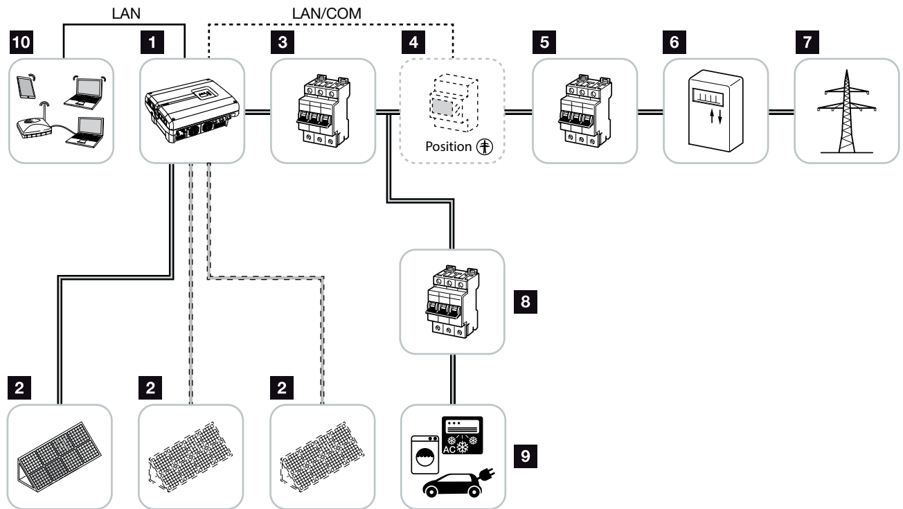
Fig. 8: Solcelleanlæg 3-faset
