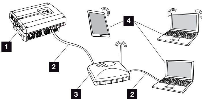
Fig. 47: Forbind vekselstrømsomformer og computer via en router
