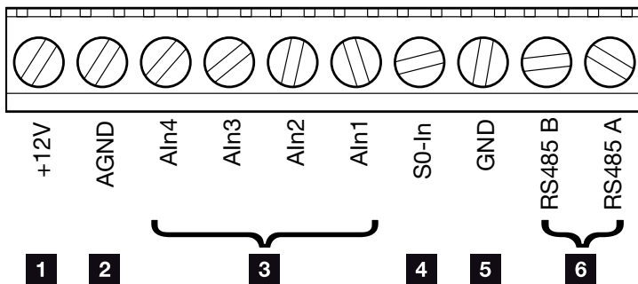
Fig. 33: Opbygning for tilslutningsklemmen 10-polet
