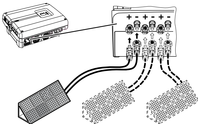
Fig. 30: Oversigt over DC-tilslutninger
