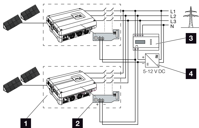
Fig. 25: Funktion koblingskontakt
