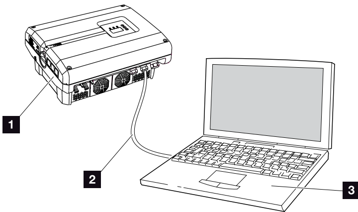
Fig. 45: Forbind vekselstrømsomformer og computer med ethernet-kabel
