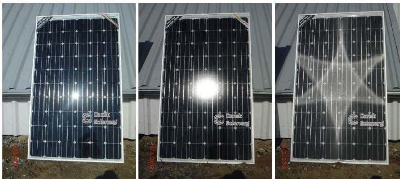
Fig.5 Glassets overfladeruhed er stigende fra venstre mod højre. Ulempen ved den høje ruhed er at snavs lettere sætter sig fast på glasset. [RHEM antireflektive solcellepaneler, Dansk Solenergi]
