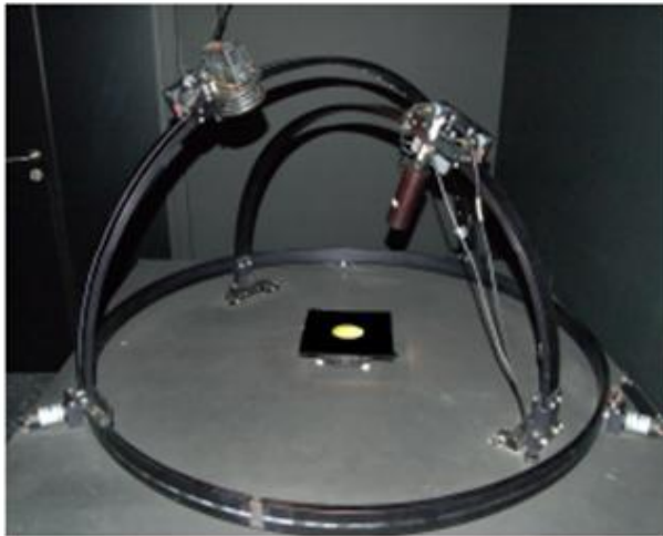
Fig.3 Eksempel på goniometer konstruktion, testemne i centrum http://www.biw.kuleuven.be/m3-biores/geomatics.htm
